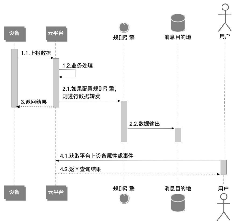
图11 设备上报属性或事件流程
