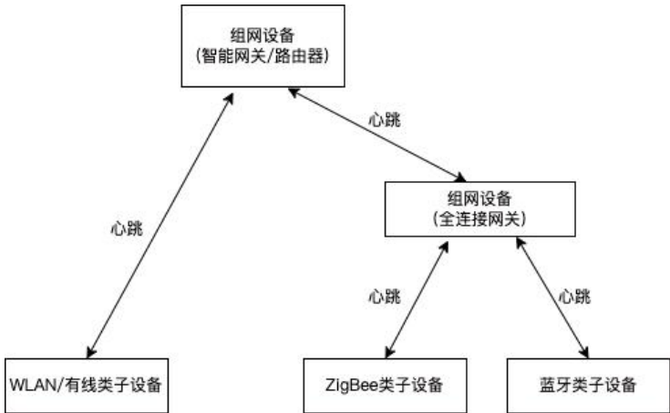
图9 局域网内设备间的心跳交互示意图
