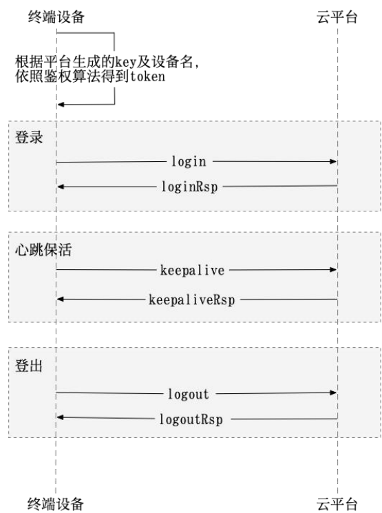
图8 设备接入流程
