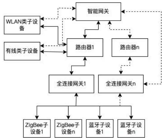
图3 局域网内互通控制方案网络架构
