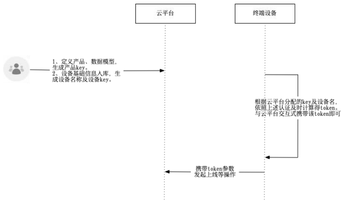
图7 认证流程和接口
