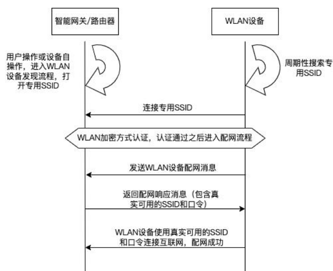
图4 WLAN设备发现和配网流程
