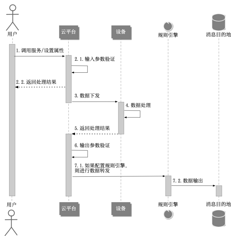
图14 异步服务调用流程
