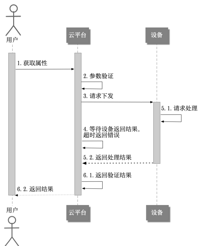
图12 设备属性获取流程
