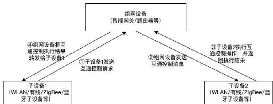
图10 局域网内子设备间的互通控制流程
