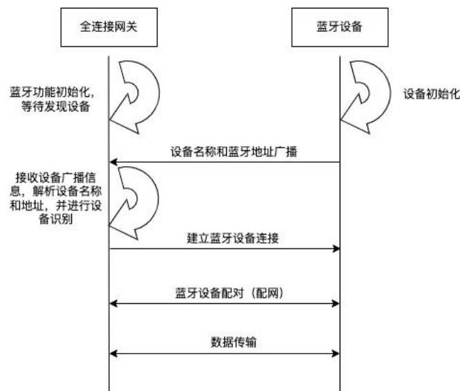
图5 蓝牙设备发现和配网流程
