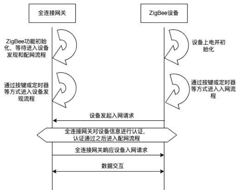
图6 Zigbee设备发现和配网流程
