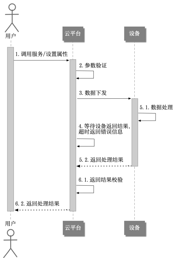
图13 同步服务调用流程
