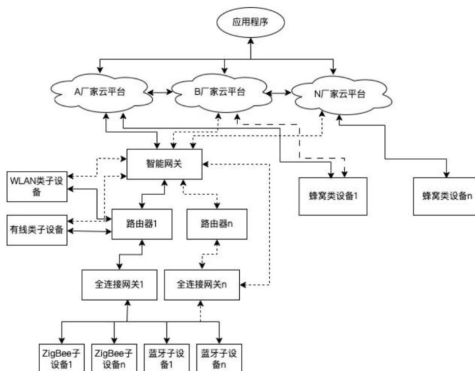
图2 端云互通控制网络架构
